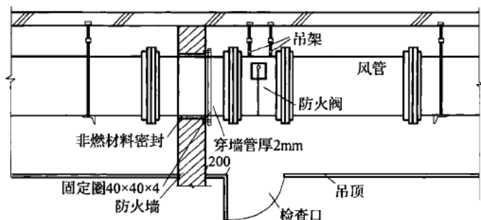
图 10 防火阀检修口设置示意图
