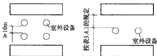
图 1 有室外设备时的防火间距
